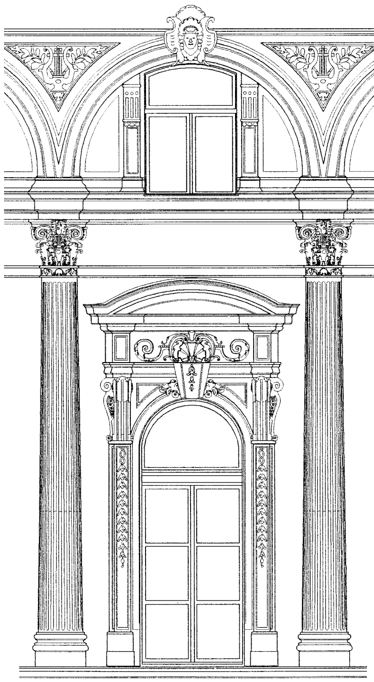
Detalj fotogrametrijske snimke pročelja sjeverne zgrade Hrvatskoga glazbenog zavoda.
